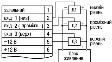
Рисунок 5.5 – Схема підключення активних датчиків Д1...Д3 із живленням їх від зовнішнього джерела
