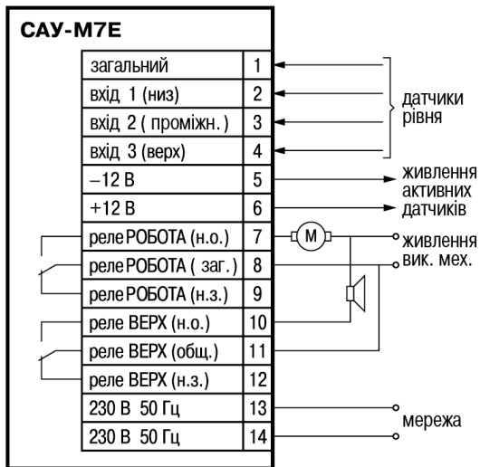
Рисунок 5.2 – Загальна схема підключення САУ-М7Е
