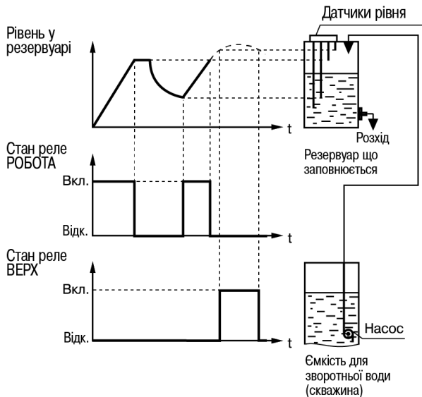
Рисунок 6.3 – Заповнення резервуара за гістерезисним законом
