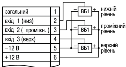
Рисунок 5.4 – Схема підключення ємнісних перемикачів
