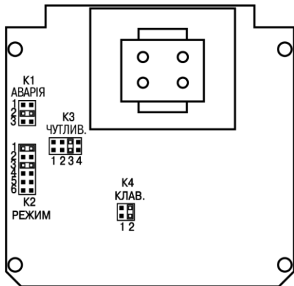
Рисунок 7.1 – Схема розташування комутаторів
