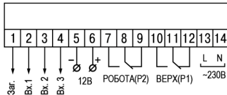
Рисунок 5.1 – Призначення клемника
