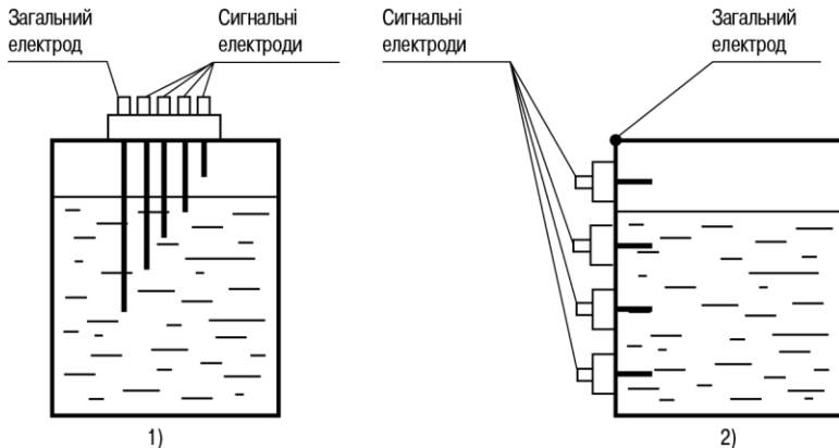
Рисунок 6.2 – Установлення електродів у неметалевий (1) і металевий (2) резервуари
