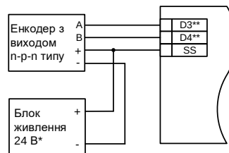
Рисунок 9 – Підключення енкодерів n-p-n типу
