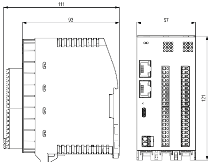
Рисунок 1 – Габаритні розміри пристрою
