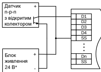
Рисунок 7 – Підключення датчиків n-p-n типу з відкритим колектором
