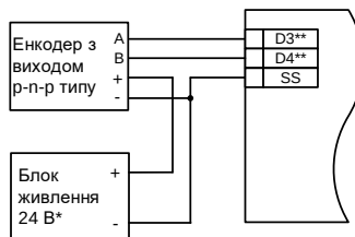
Рисунок 8 – Підключення енкодерів p-n-p типу
