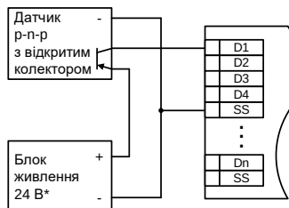
Рисунок 6 – Підключення датчиків p-n-p типу з відкритим колектором
