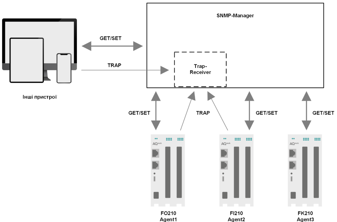
Рисунок 6.2 – Структурна схема обміну за протоколом SNMP
