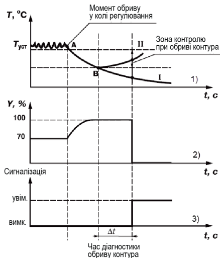
Рисунок 7.14 – Спрацювання діагностики обриву
