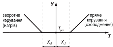
Рисунок 7.9 – Регулювання сигналу в зоні нечутливості
