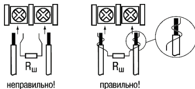
Рисунок 5.7 – Підключення датчиків з виходом у вигляді струму або напруги УВАГА
