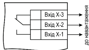
Рисунок 5.11 – Схема підключення навантаження до ВП типу Р
