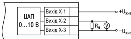
Рисунок 5.18 – Схема підключення навантаження до ВП типу У
