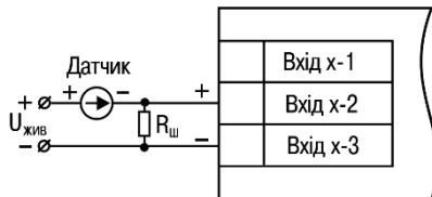
Рисунок 5.9 – Схема підключення пасивного датчика зі струмовим виходом 0...5 мА або 0(4)...20 мА R_{ш} = 100 \pm 0,1 \text{ Ом}
