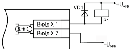
Рисунок 5.12 – Схема підключення навантаження до ВП1 типу К
