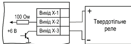
Рисунок 5.13 – Схема підключення навантаження до ВП типу Т
