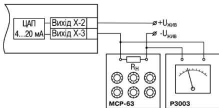
Рисунок 8.7 – Підключення ВП1 типу І ( R_H = 500\text{ }\Omega )
