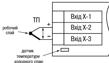
Рисунок 5.6 – Схема підключення термопари
