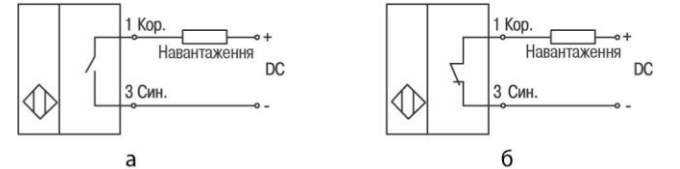
Рисунок 9 – Схема підключення двоводових датчиків:
