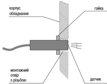
Рисунок 3 – Установлення датчика, що передбачає занурення
