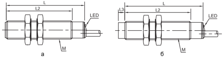
Рисунок 1 – Габаритні розміри датчика: а – що передбачає занурення; б – що не передбачає занурення
