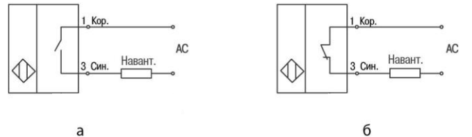
Рисунок 10 – Схема підключення двоводових датчиків змінного струму:
