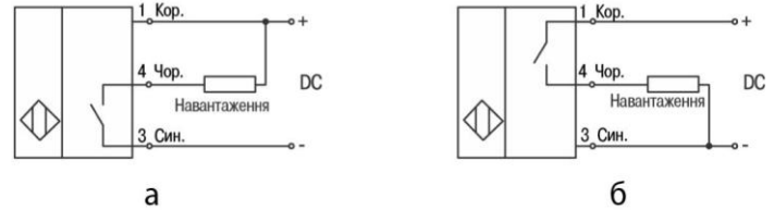
Рисунок 6 – Схема підключення трипроводових NO-датчиків:
