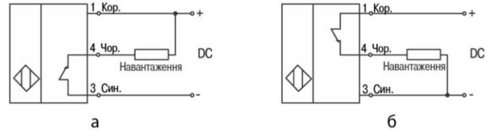
Рисунок 7 – Схема підключення трипроводових NC-датчиків:
