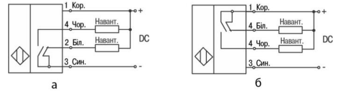
Рисунок 8 – Схема підключення чотириводових NO+NC-датчиків:
