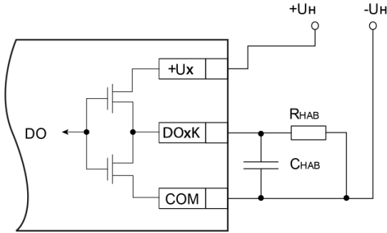
Рисунок 4 – Схема підключення навантаження у режимі вмикання «верхній і нижній ключі»
