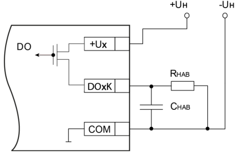
Рисунок 3 – Схема підключення навантаження у режимі вмикання «верхній ключ»
