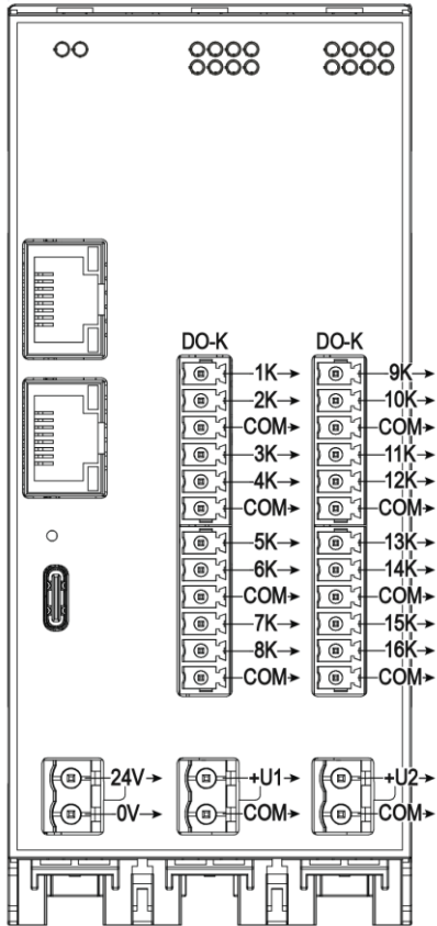
Рисунок 2 – Призначення контактів клемника FO210-16FK
