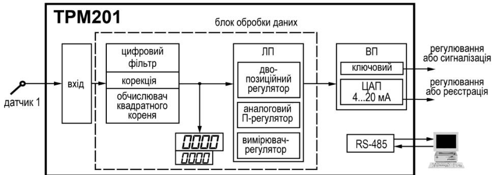
Рисунку 6.1 – Функціональна схема пристрою
