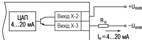
Рисунок 5.15 – Підключення до ВП типу I
