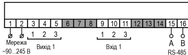
Рисунок 5.2 – Загальна схема підключення TRM201-N, -Щ1 і -Щ2
