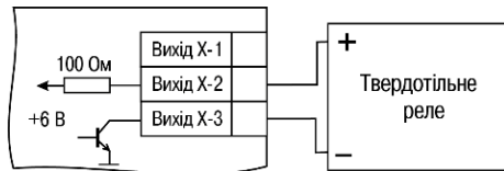
Рисунок 5.12 – Схема підключення навантаження до ВП типу Т
