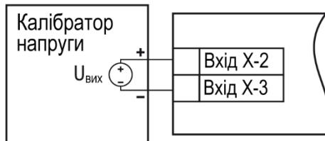
Рисунок 8.3 – Підключення калібрування напруги
