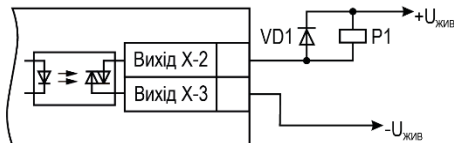
Рисунок 5.11 – Схема підключення навантаження до ВП типу К
