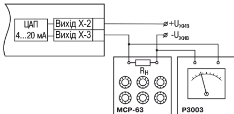
Рисунок 8.7 – Підключення ВП1 типу І ( R_H = 500 \text{ Ом} )
