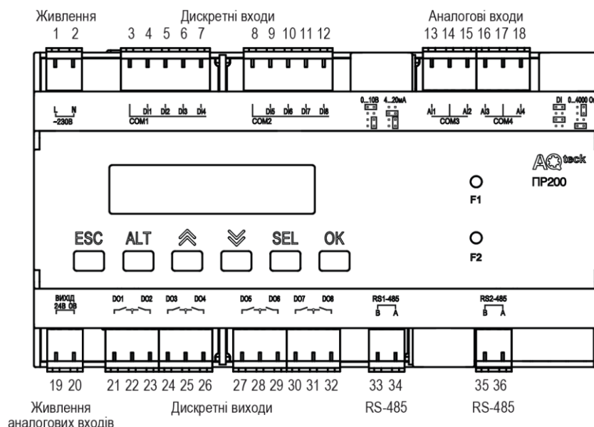
Рисунок А.2 – Розташування контактів ПР200-230.3.2.0
