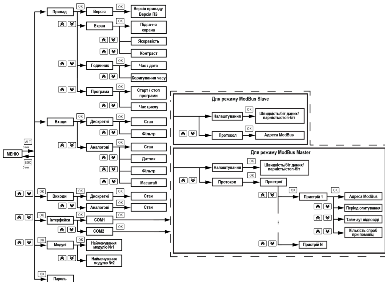
Рисунок 7.2 – Структура системного меню
