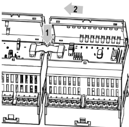
Рисунок 5.13 – Укладання шлейфа в поглиблення
