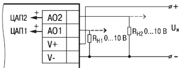
Рисунок 5.12 – Схема підключення навантаження до ВЕ типу «У»
