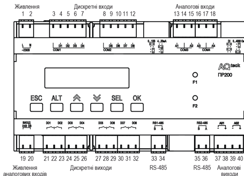
Рисунок А.1 – Розташування контактів PR200-230.2.2.0
