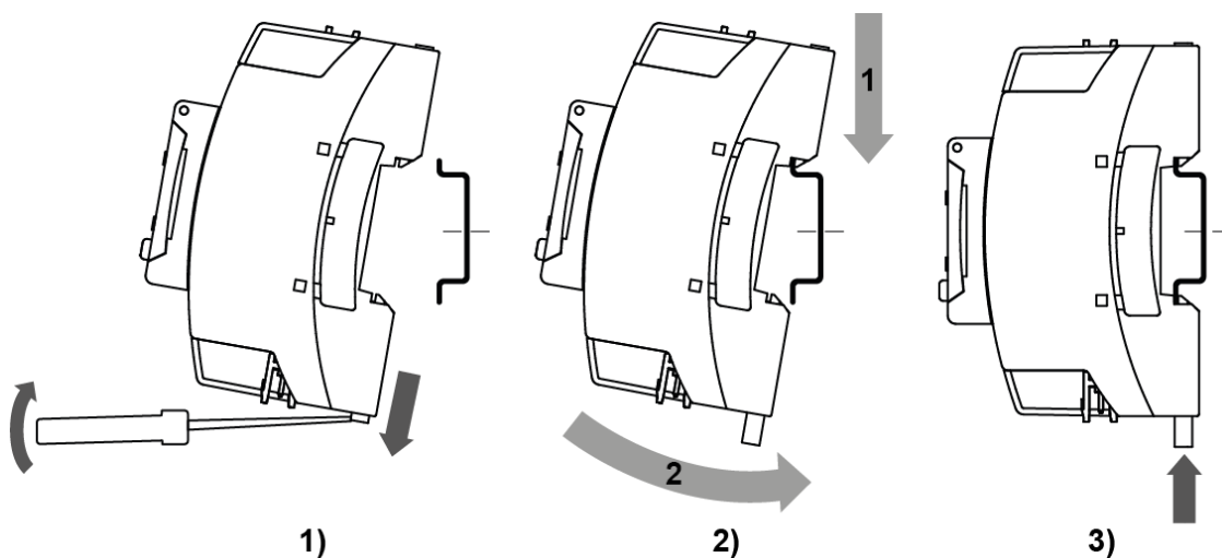
Рисунок 4.1 – Монтаж і демонтаж пристрою
