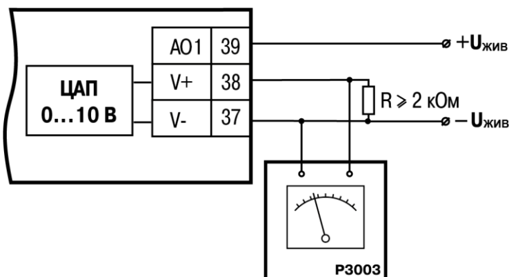
Рисунок 8.10 – Схема підключення навантаження до ВЕ типу «У»
