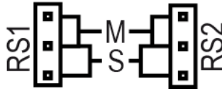
Рисунок 6.8 – Положення перемичок підтягувальних резисторів
