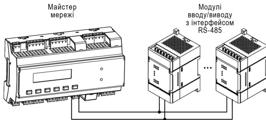
Рисунок 5.16 – Типова схема підключення для PR200 в режимі Master
