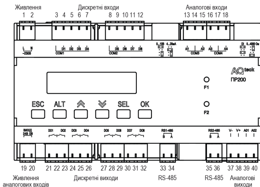
Рисунок А.3 – Розташування контактів PR200-230.4.2.0
