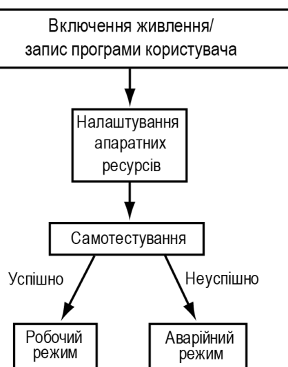
Рисунок 6.6 – Алгоритм запуску пристрою
