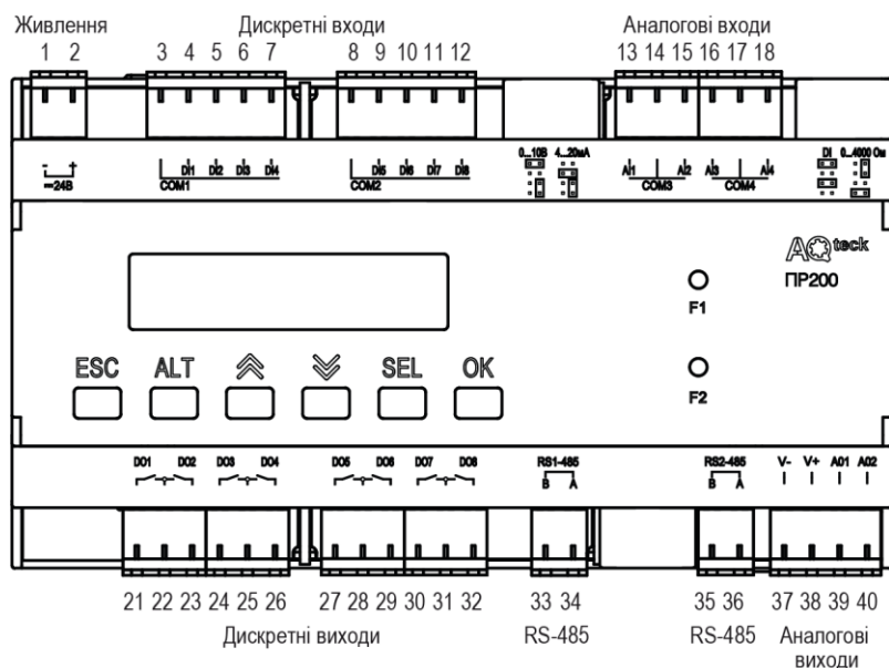
Рисунок А.6 – Розташування контактів PR200-24.4.2.0
