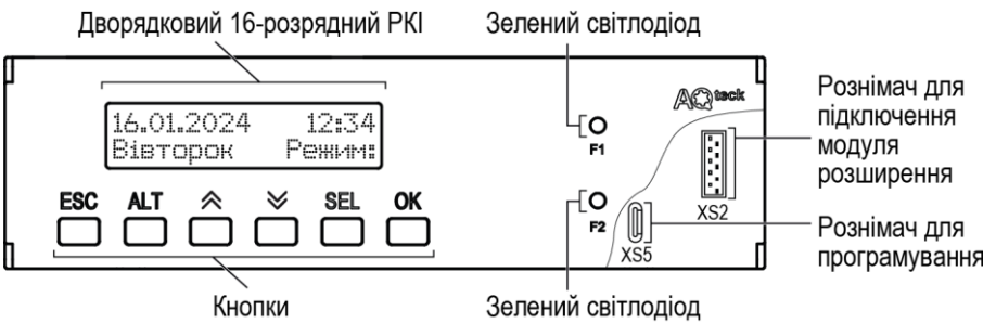
Рисунок 7.1 – Лицьова панель пристрою
