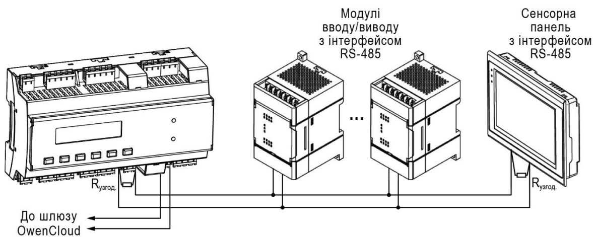
Рисунок 5.17 – Змішана схема підключення
