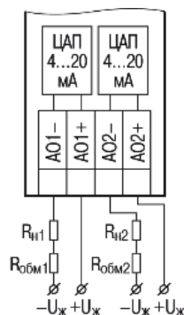
Рисунок 5.10 – Схема підключення навантаження до ВЕ типу «И»
