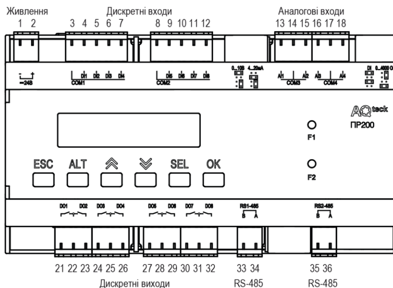
Рисунок А.5 – Розташування контактів ПР200-24.3.2.0
