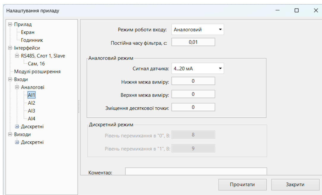
Рисунок 6.1 – Меню налаштування пристрою
