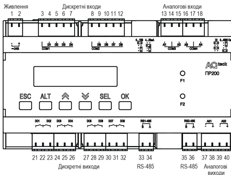
Рисунок А.4 – Розташування контактів ПР200-24.2.2.0
