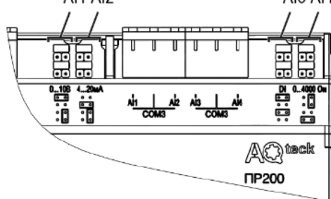
Рисунок 6.3 – Схема розташування перемичок
