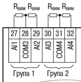
Рисунок 5.6 – Схема підключення резистивного датчика з діапазоном 0...4000 Ом
