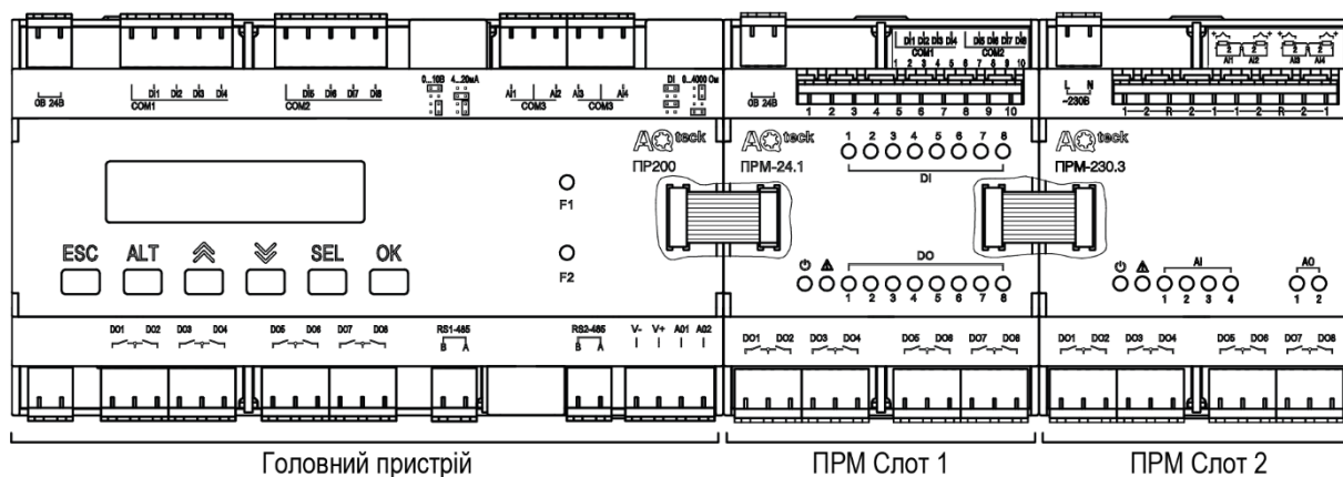
Рисунок 5.14 – Розташування модулів розширення на шині
