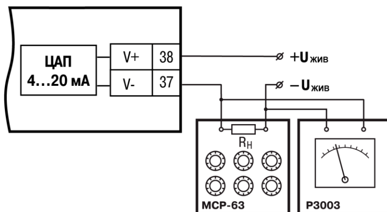
Рисунок 8.8 – Схема підключення до ВЕ типу «И» ( R_H = 500 \text{ Ом} )
