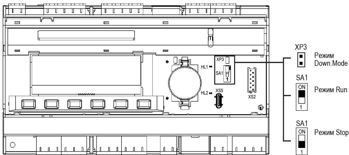
Рисунок 6.7 – Вид на верхню плату з відкинутою кришкою
