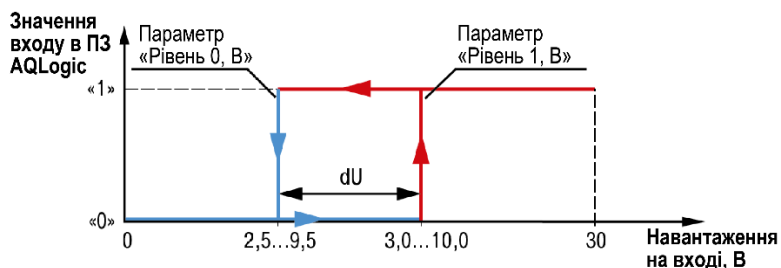
Рисунок 6.5 – Робота універсального входу в дискретному режимі
