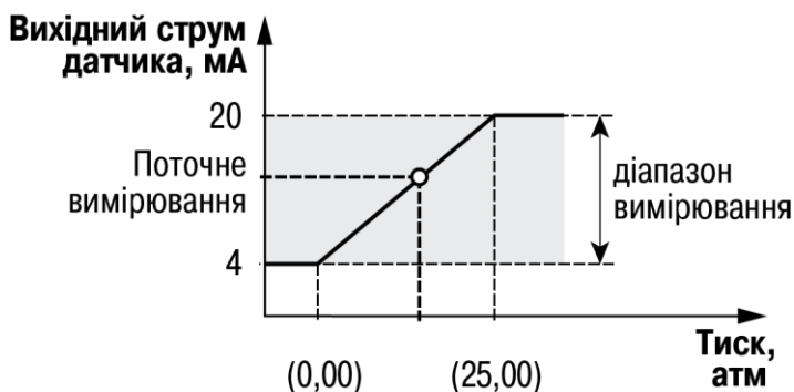
Рисунок 6.4 – Приклад задавання діапазону вимірювання
