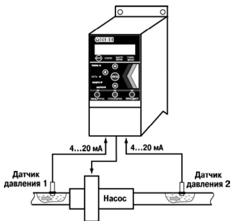
Рисунок 4.6 - Схема установки
