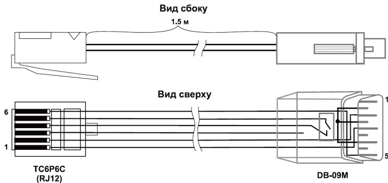
Рисунок Б.3 – Схема “Модемный кабель ПЛК1XX”
