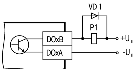
б) для выходов DO5 – DO8
