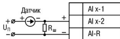
Рисунок Б.5 – Подключение активного датчика с токовым выходом 0...5 мА или 0(4)...20 мА ( R_{\text{ш}} = 100,0 \text{ Ом} \pm 0,1\% )
