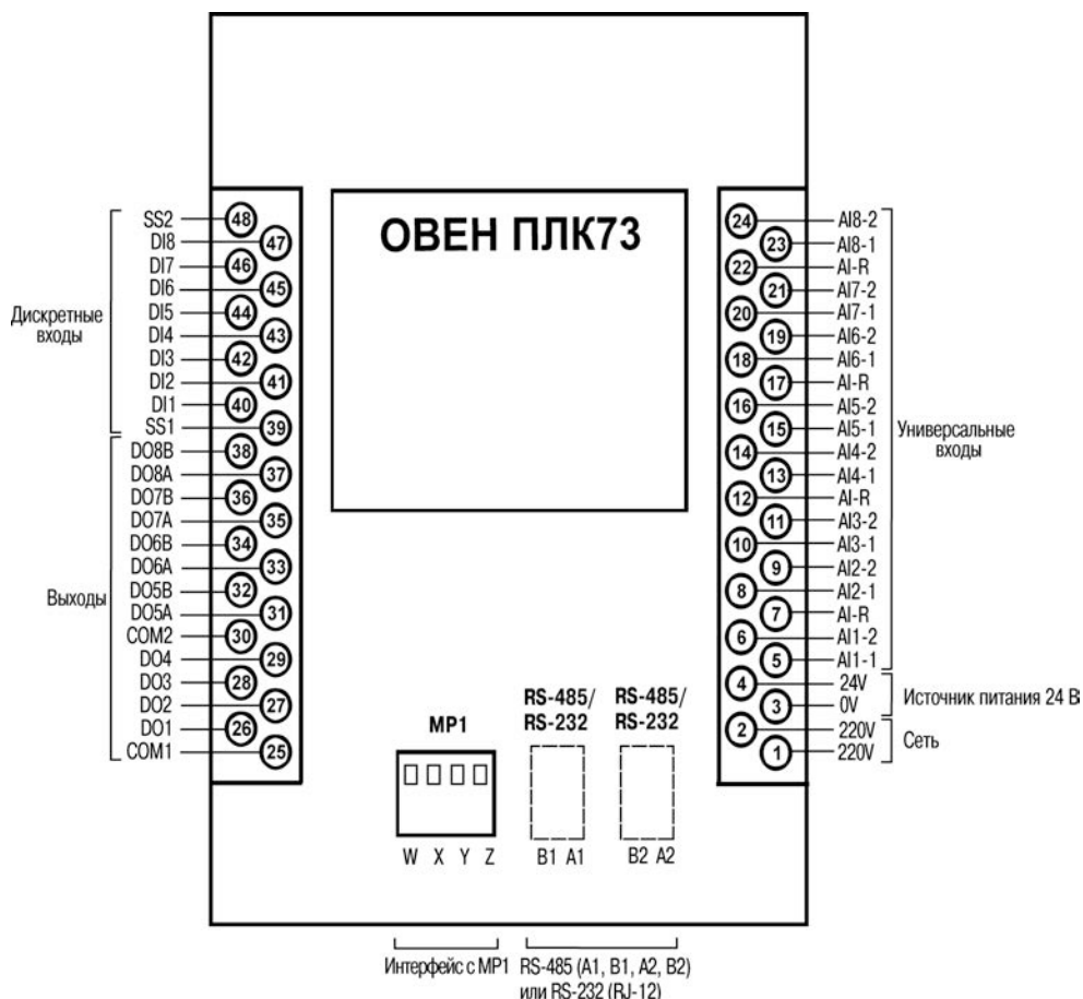
Рисунок Б.15 – Схема расположения и назначения клемм контроллера (вид на заднюю стенку корпуса)
