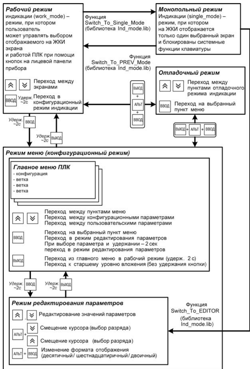
Рисунок 7.1 – Диаграмма переходов между режимами индикации контроллера
