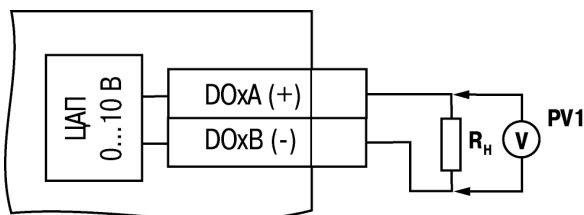
Рисунок Б.7 – Схема подключения нагрузки к ВЭ типа «У». R_{\text{н}} > 2 \text{ кОм}
