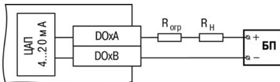
Рисунок Б.8 – Схема подключения нагрузки к ВЭ типа «И»
