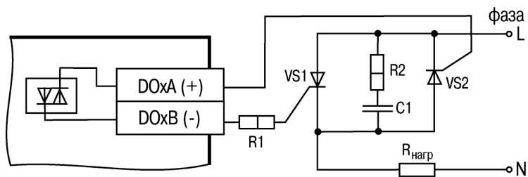
Рисунок Б.12 – Схема подключения нагрузки к ВЭ типа «С» двух тиристоров, подключенных встречно-параллельно ( R2=47 \dots 68 \text{ Ом} , C1=0.1 \text{ мкФ} \times 630 \text{ В} )
