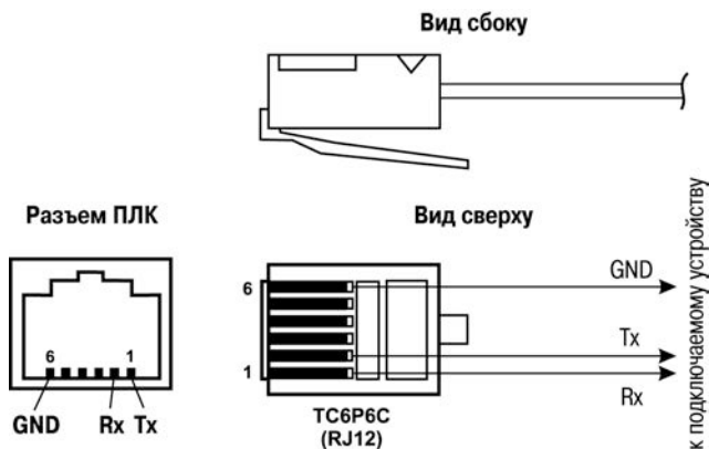
Рисунок В.3 – Схема кабеля для подключения контроллера к порту RS-232
