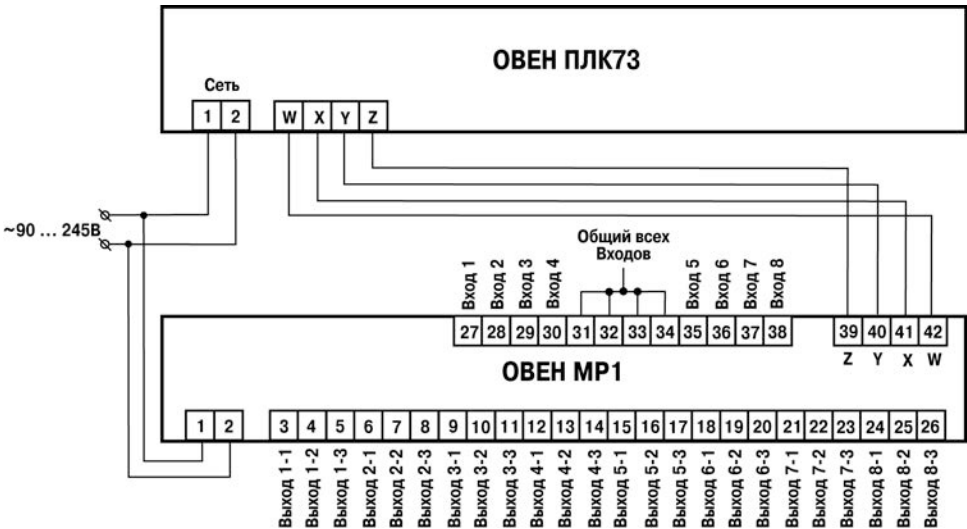
Рисунок Б.14 – Схема подключения модуля ОВЕН МР1 к ОВЕН ПЛК73
