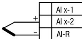
Рисунок Б.6. – Схема подключения термопары (термоэлектрического преобразователя)
