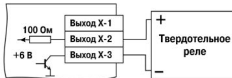
Рисунок Б.8 – Схема подключения к ВУ вида Т
