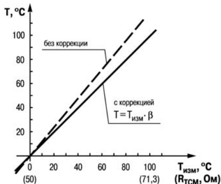
Рисунок 3.4 – Коррекция «наклон характеристики»
