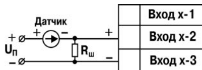
Рисунок Б.12 – Схема подключения активного датчика с токовым выходом от 0 до 5, от 0 до 20, от 4 до 20 мА
