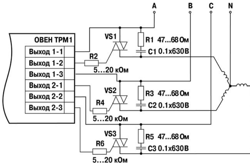
Рисунок Б.5 – Схема подключения трех симисторных оптопар (ОБЕН TPM1-Х.У.С3)
