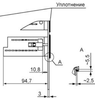
Рисунок А.7 – Прибор в корпусе Щ2, установленный в щит толщиной 3 мм
