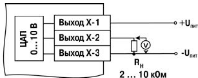
Рисунок Б.7 – Схема подключения нагрузки к ВУ вида У
