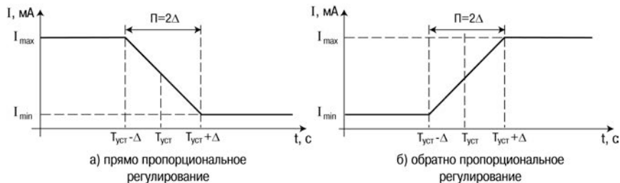
Рисунок 3.13 – Принцип формирования управляющего тока П-регулятора
