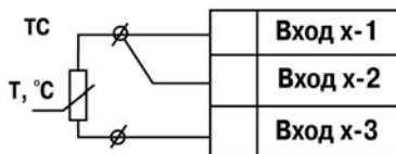
Рисунок Б.9 – Схема подключения термопреобразователя сопротивления
