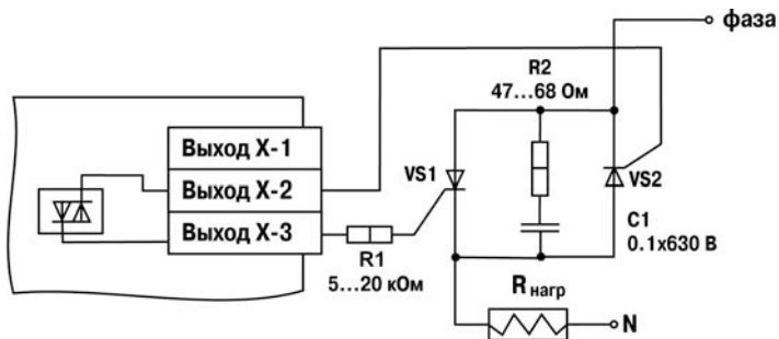
Рисунок Б.4 – Схема подключения к ВУ вида С двух тиристоров, включенных встречно-параллельно
