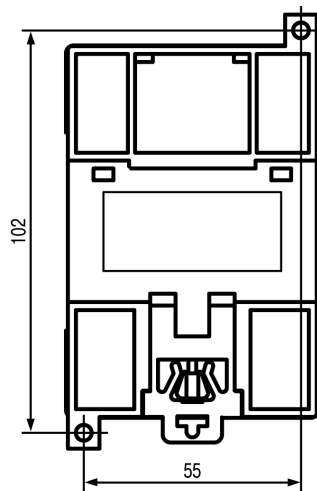
Рисунок А.2 – Установочный чертеж
