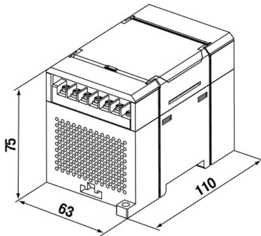
Рисунок А.1 – Габаритный чертеж прибора
