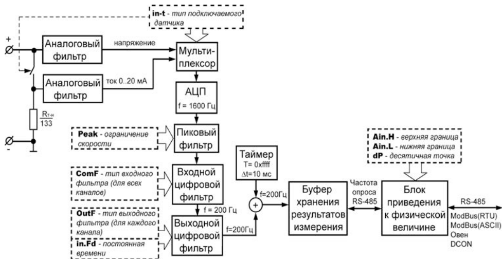
Рисунок 3.1 – Структурная схема прибора
