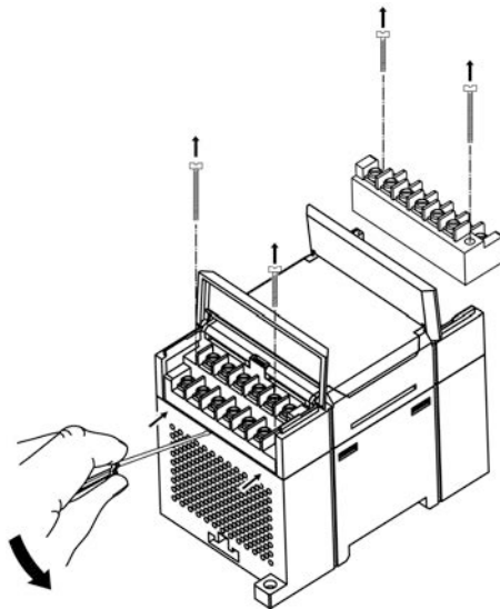
Рисунок Д.1 – Отделение клеммной колодки от прибора ОВЕН МВ110-224.1ТД
