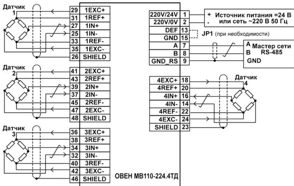
Рисунок 6.2 – Подключение к ОБЕИ MB110-224.4ТД внешних устройств с применением шестипроводной схемы подключения к датчику и без использования заземления
