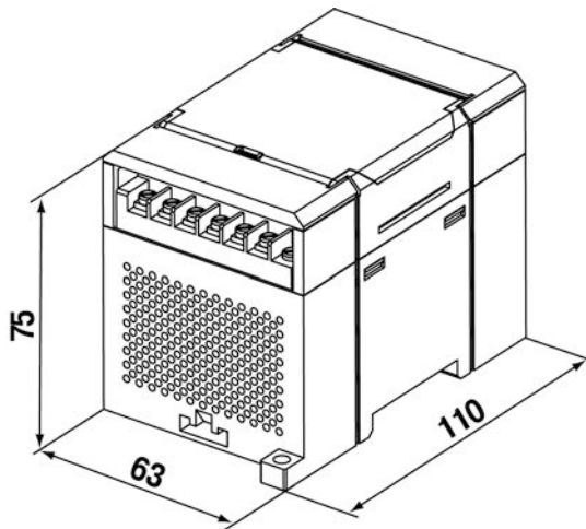
Рисунок А.1 – Габаритный чертеж ОВЕН МВ110-224.1ТД
