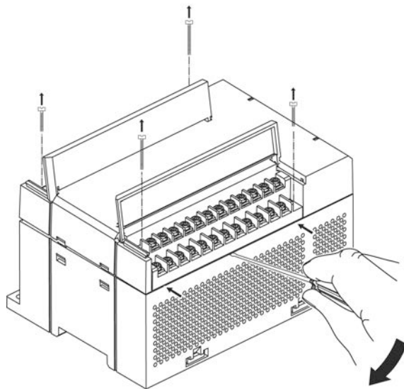
Рисунок Д.2 – Отделение клеммной колодки от прибора ОВЕН МВ110-224.4ТД
