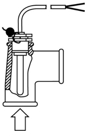
Рисунок 5.2 - Пломбировка КДТС054
