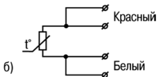
Рисунок В.1 – Схема подключения КДТС с кабельными выводами: а) двухпроводная схема, б) четырехпроводная схема
