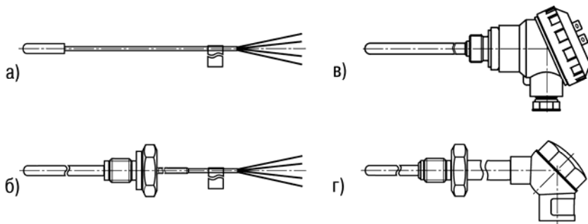
Рисунок 3.1 – Варианты исполнения КДТС: а) погружной без штуцера, б) погружной со штуцером, в) с металлической коммутационной головкой и приварным штуцером; г) с пластиковой коммутационной головкой и подвижным штуцером.
