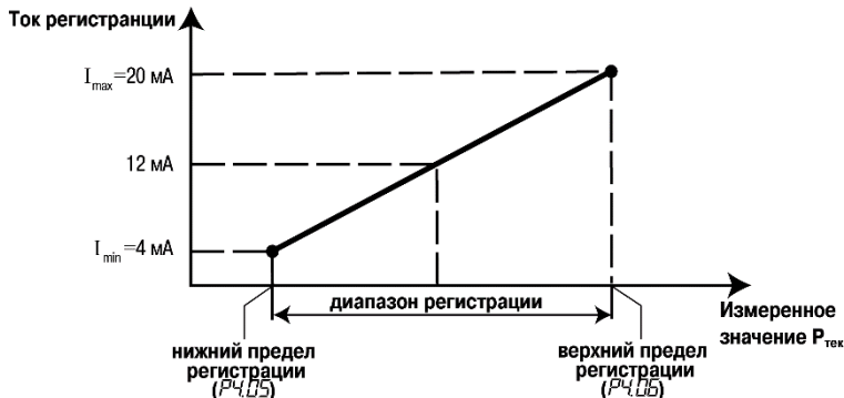
Рисунок 5.4 – Принцип формирования тока регистрации
