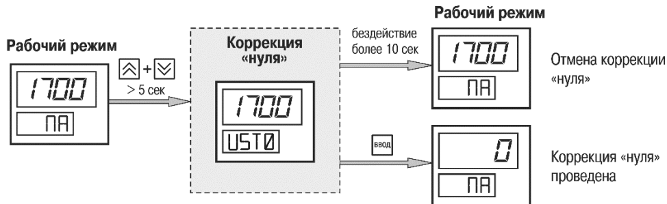
Рисунок Д.2 – Пользовательская коррекция «нуля»
