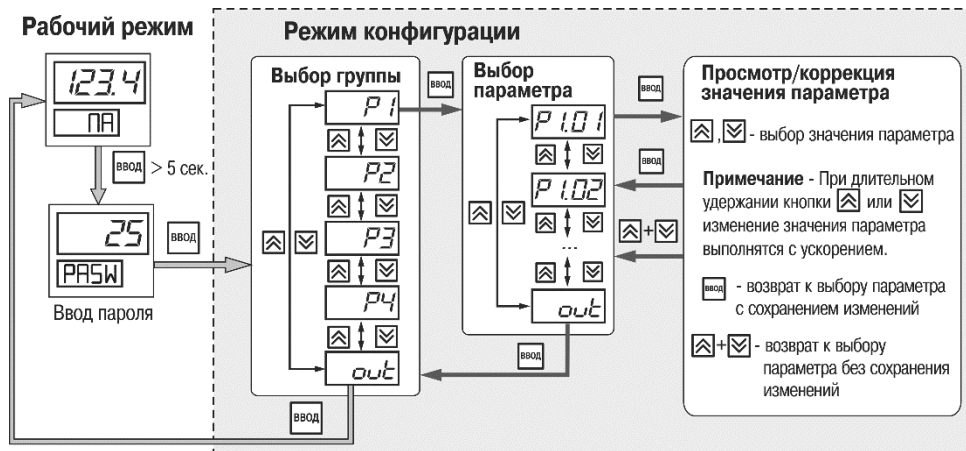
Рисунок 5.1 – Режим конфигурации
