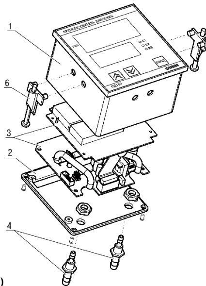
Рисунок 4.2 – Конструкция преобразователя ПД150-ДД настенного (а) и щитового (б) крепления
