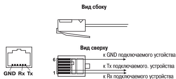
Распиновка кабеля KC1.
