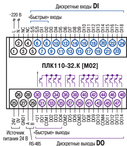
Схема расположения и назначение клемм ПЛК110-220.32.К [M02]
