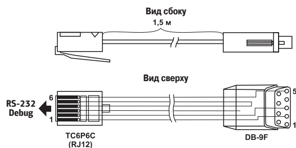
Схема кабеля для программирования KC1, входящего в комплект поставки.
