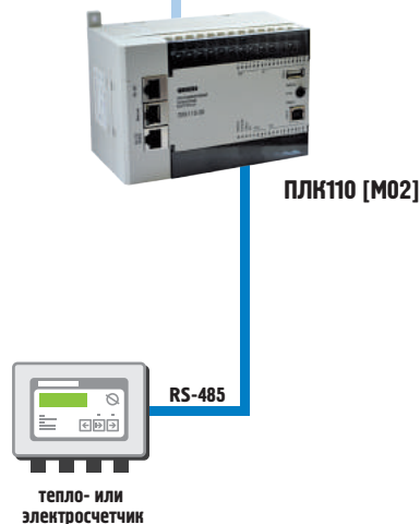
Опрос тепло- и электросчетчиков и передача данных в сеть верхнего уровня по Ethernet
