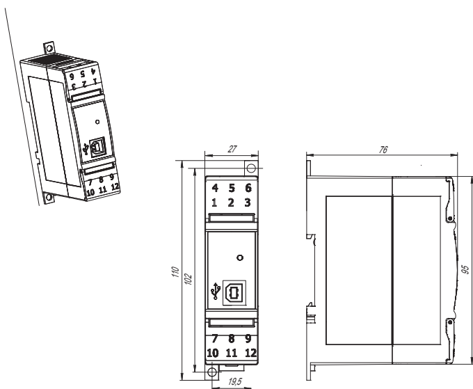
Д1,5 — корпус для крепления на DIN-рейку габаритные размеры: 27х110х76 мм степень защиты со стороны передней панели IP20
