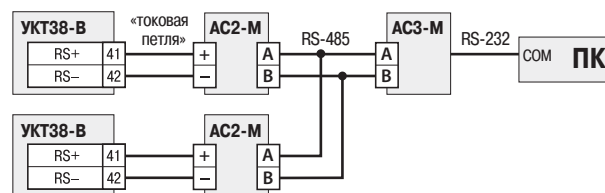
Схема подключения приборов УКТ38-В к ПК через преобразователи AC2-M и AC3-M
