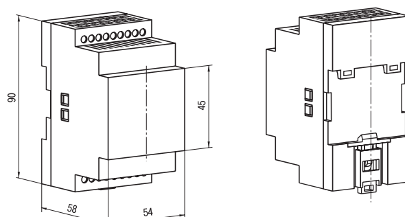
Д3 — корпус для крепления на DIN-рейку 35 мм, габаритные размеры: 54х90х58 мм степень защиты со стороны передней панели IP20
