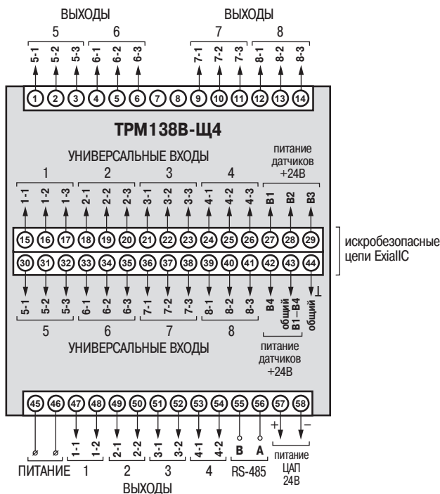
Схема расположения и назначения клемм ТРМ138В в корпусе Щ4
