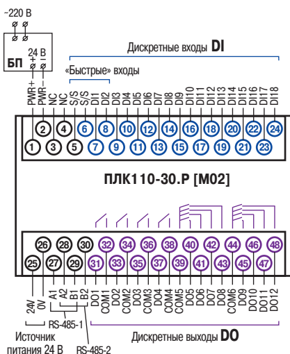
Схема расположения и назначение клемм ПЛК110-24.30.Р [M02]
