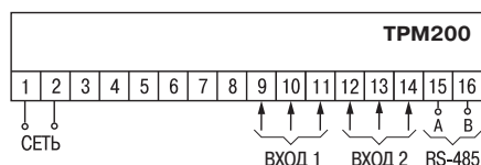
Схема расположения и назначения клемм TPM200
