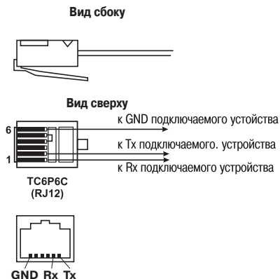
Распиновка кабеля KC1.
