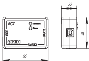
Габаритные размеры AC7
