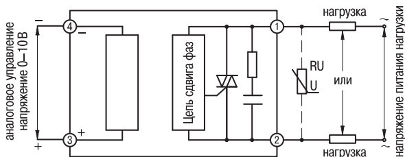
Схема включения серии HD-xx22.10U
