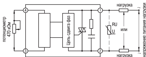
Схема включения серии HD-xx44.VA
