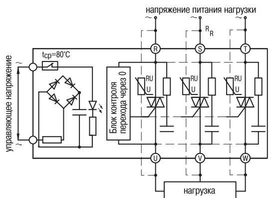
Схема включения серии HT-xx44.ZA2 (выходы – семисторы (TRIAC))
