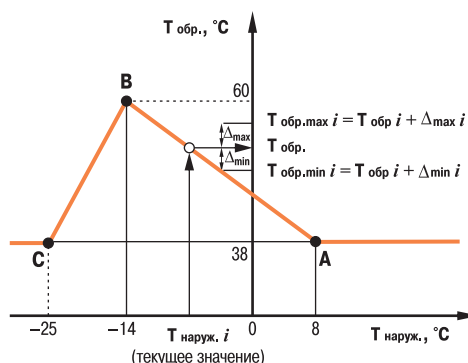
Пример графика температуры обратной воды — T_{\text{обр.}} = f(T_{\text{нар.}})
