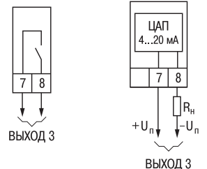
ВЭ3 типа P (э/м реле)
