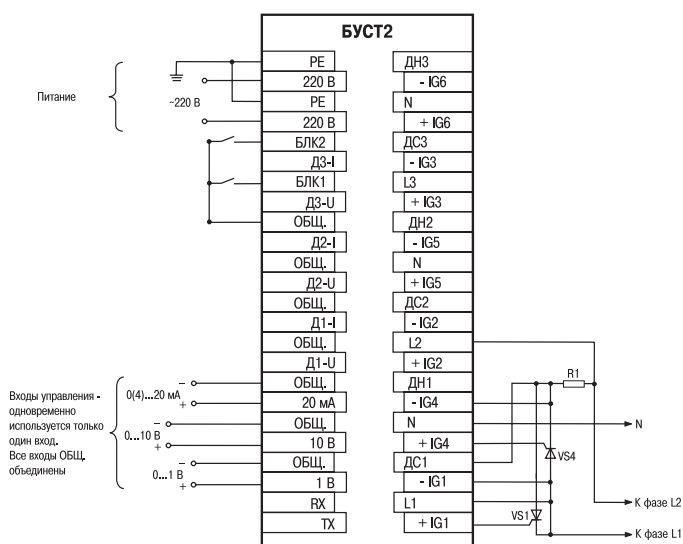
Схема соединения для типа подключения нагрузки «одна фаза, 380 В»
