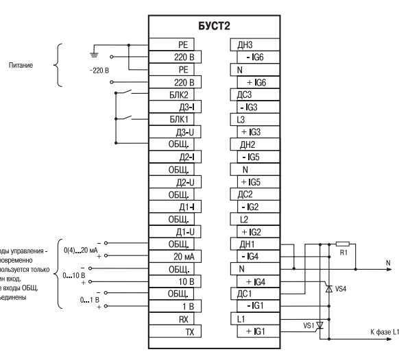
Схема соединения для типа подключения нагрузки «одна фаза, 220 В»
