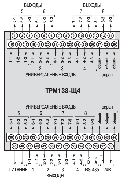
Схема расположения и назначения клемм ТРМ138 в корпусе Щ4
