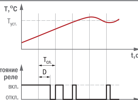
Выходной сигнал регулятора и временная диаграмма выходного реле при ШИМ-управлении нагревателем
