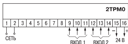
Схема расположения и назначения клемм ТРМ200
