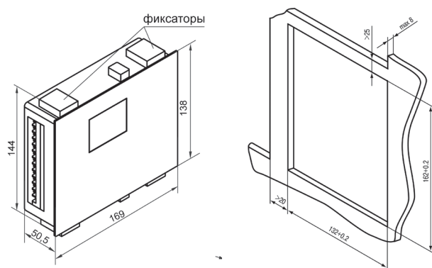
Щ7 — корпус щитового крепления габаритные размеры: 169х138х50 мм, степень защиты со стороны передней панели IP54
