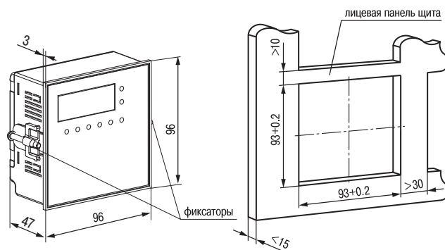
Щ11 — корпус щитового крепления габаритные размеры: 96х96х49 мм, степень защиты со стороны передней панели IP54
