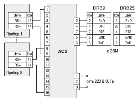
Схема подключения прибора МПР51
