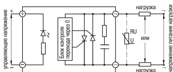
Схема включения серии BDH-xx44.ZD3
