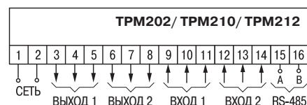
Схема расположения и назначения клемм TPM202, TPM210, TPM212
