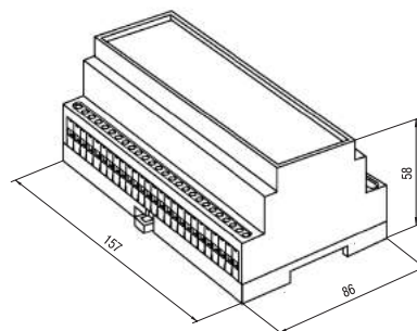
Д9 — корпус для крепления на DIN-рейку 35 мм, габаритные размеры: 157х86х58 мм, степень защиты со стороны передней панели IP20
