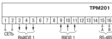
Схема расположения и назначения клемм TPM201
