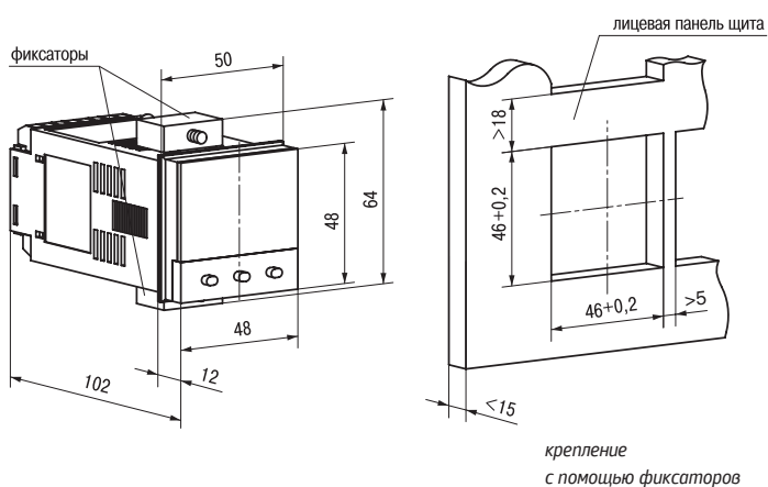
Щ5 — корпус щитового крепления габаритные размеры: 48х48х102 мм степень защиты со стороны передней панели IP54
