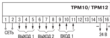
Схема расположения и назначения клемм ТРМ10, ТРМ12
