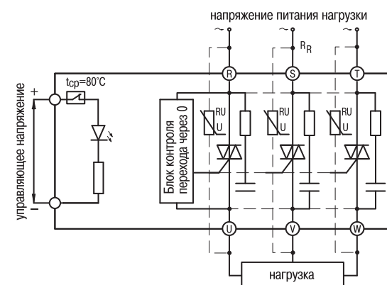
Схема включения серии HT-xx44.ZD3 (выходы – семисторы (TRIAC))
