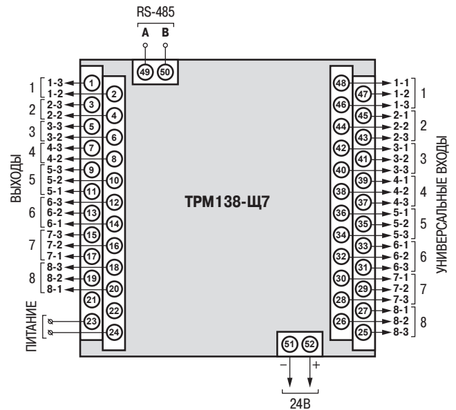
Схема расположения и назначения клемм ТРМ138 в корпусе Щ7
