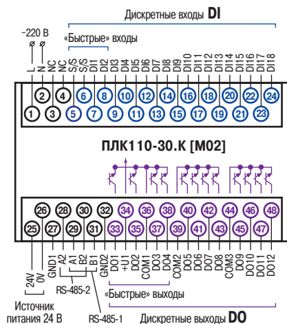
Схема расположения и назначение клемм ПЛК110-220.30.К [M02]
