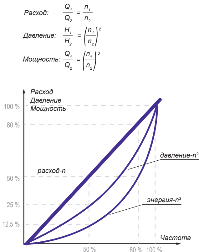
Рис. 1. Законы пропорциональности.
