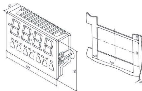
Щ8 — корпус щитового крепления габаритные размеры: 144х96х43 мм, степень защиты: со стороны передней панели IP54 со стороны цилиндрической части корпуса IP20
