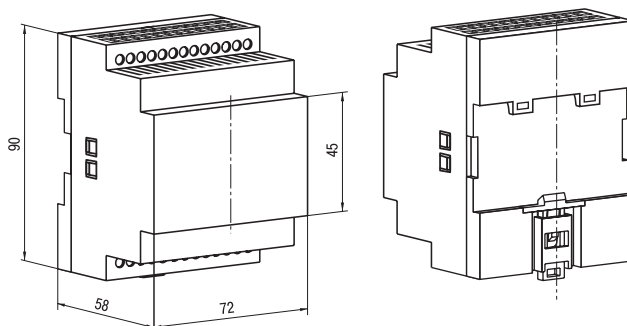
Д4 — корпус для крепления на DIN-рейку 35 мм габаритные размеры: 72х90х58 мм, степень защиты со стороны передней панели IP20
