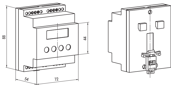
Д — корпус для крепления на DIN-рейку габаритные размеры: 72х88х54 мм степень защиты со стороны передней панели IP20
