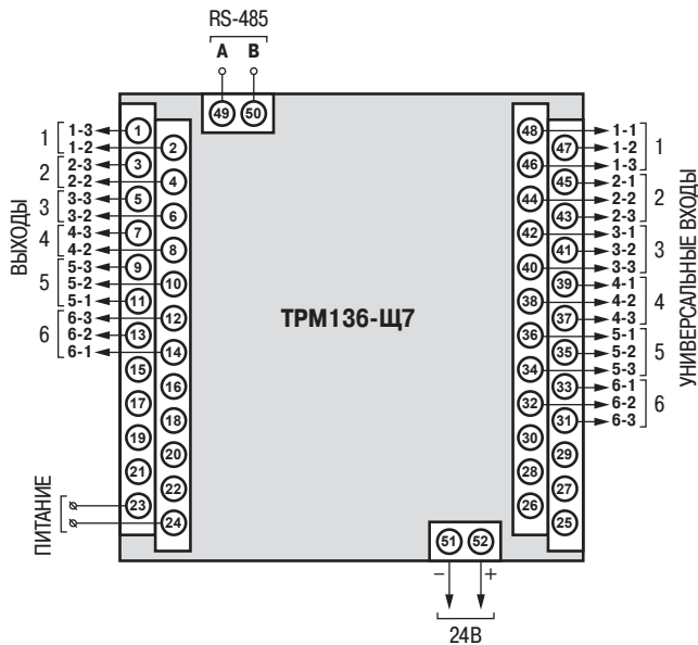
Схема расположения и назначения клемм ТРМ136 в корпусе Щ7
