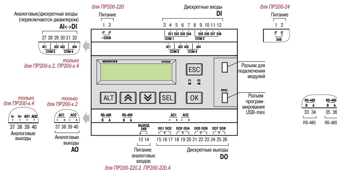
Схема расположения и назначение клемм ПР200
