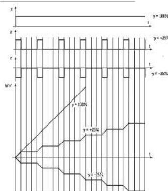
График сигналов на выходе ШИМ и ИМ при управлении средней скоростью регулирующего воздействия Y'
