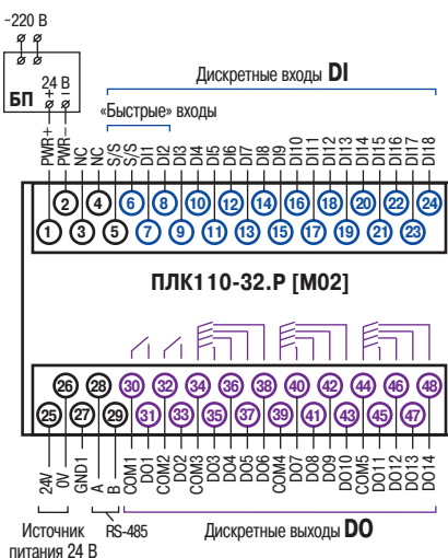
Схема расположения и назначение клемм ПЛК110-24.32.Р [M02]
