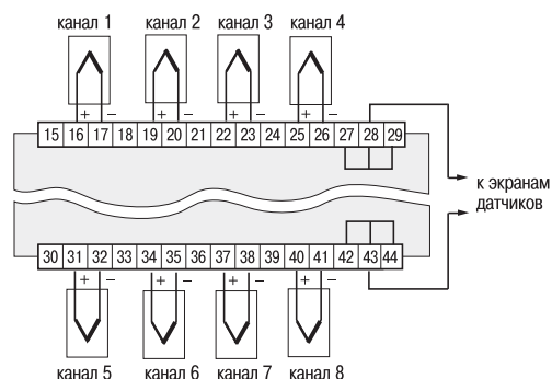
Схема подключения приборов модификаций УКТ38-Щ4-ТП и УКТ38-Щ4-ТПП с термоэлектрическими преобразователями
