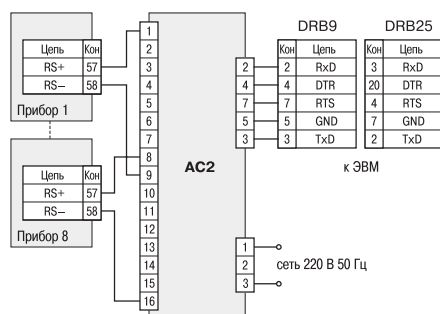
Схема подключения приборов ТРМ32, ТРМ33, УКТ38-В, УКТ38-Щ4
