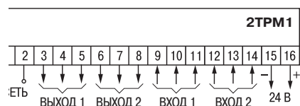
Схема расположения и назначения клемм ТРМ202
