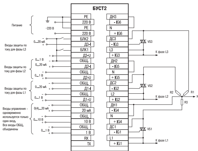
Схема соединения для типа подключения нагрузки «звезда с нейтралью и симисторами»
