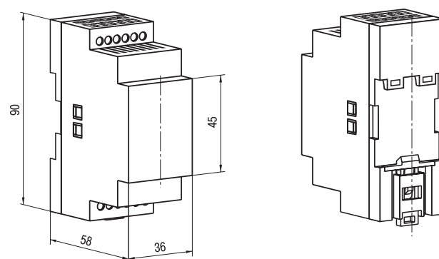
Д2 — корпус для крепления на DIN-рейку 35 мм габаритные размеры: 36х90х58 мм степень защиты со стороны передней панели IP20
