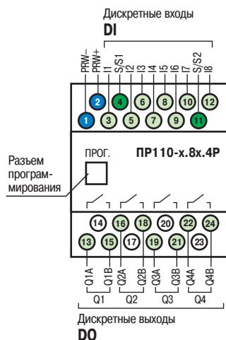
Схема расположения и назначение клемм PR110-x.8x.4P
