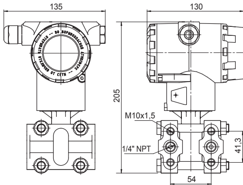
Конструктивное исполнение датчика ПД200-ДД модели 155
