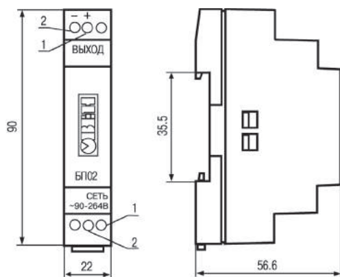
Д1 — корпус для крепления на DIN-рейку габаритные размеры: 22х90х56,6 мм степень защиты со стороны передней панели IP20
