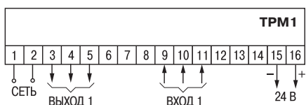
Схема расположения и назначения клемм ТРМ201
