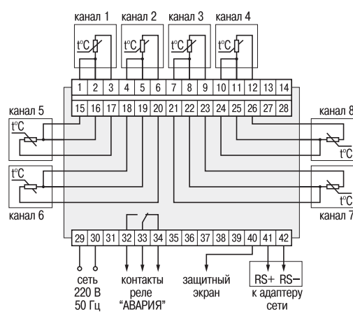
Схема подключения прибора модификаций УКТ38-В.01 и УКТ38-В.03 с термопреобразователями сопротивления типа ТСМ, ТСР
