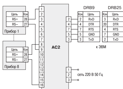
Схема подключения приборов ТРМ0-РiC, ТРМ1-РiC, ТРМ5-РiC, ТРМ10-РiC, ТРМ12-РiC
