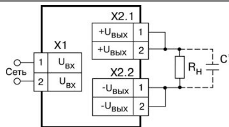
Рисунок 2 – Типовая схема подключения блока
