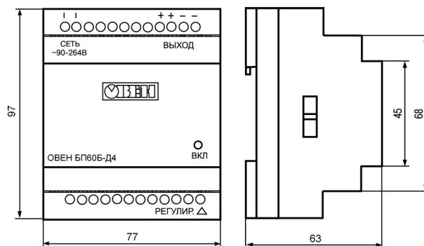
Рисунок 1 – Габаритные размеры блока
