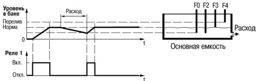
Рисунок В.17 – Графики, поясняющие работу прибора
