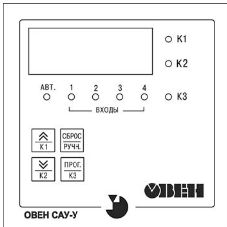
Рисунок 3.2 – Внешний вид лицевой панели прибора для корпуса щитового (Щ11) крепления
