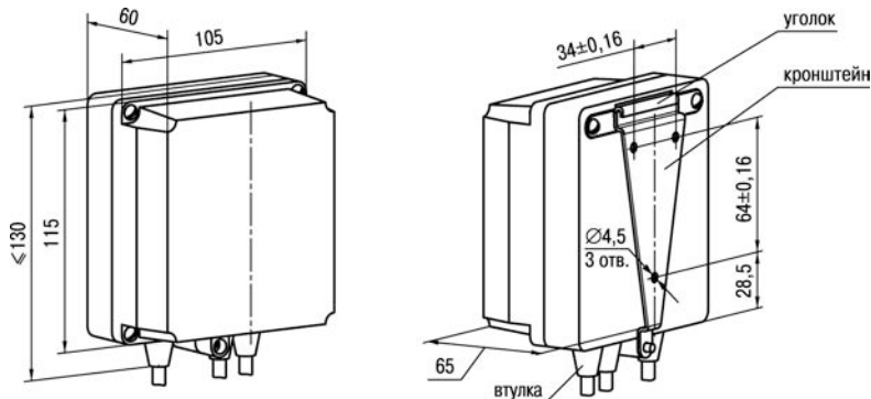
Рисунок А.1 – Прибор в корпусе типа Н (для настенного крепления)
