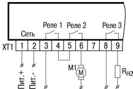
Рисунок В.16 – Подключение контактов реле 2 в ОВЕН САУ-У-Н для выполнения алгоритма 20 с защитным отключением насоса М1
