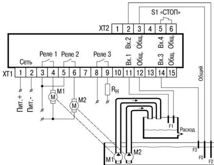
Рисунок В.14 – Схема подключения ОВЕН САУ-У-Н для выполнения алгоритма 18 M1 и M2 – насосы; F1–F3 – кондуктометрические датчики уровня; Rn – сигнализатор аварии (неисправность насоса)
