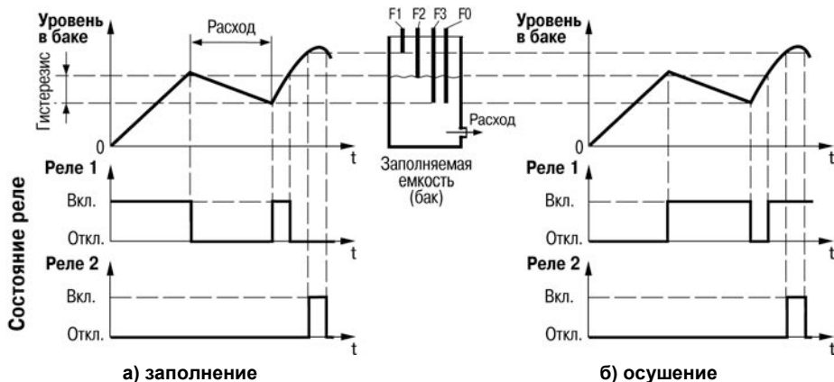
Рисунок В.2 – Графики, поясняющие работу прибора
