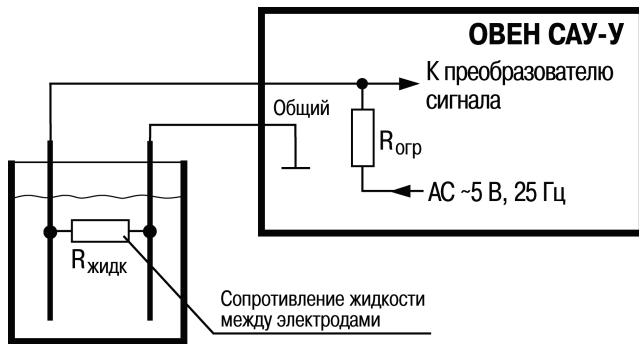
Рисунок 3.6 – Схема подключения кондуктометрического зонда
