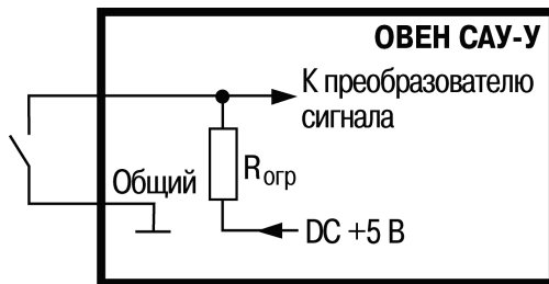
Рисунок 3.7 – Схема подключения механических контактных датчиков
