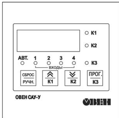
Рисунок 3.1 – Внешний вид лицевой панели прибора для корпуса настенного (Н) крепления
