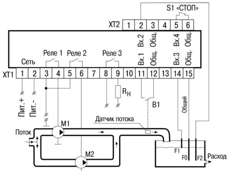
Рисунок В.8 – Схема подключения ОВЕН САУ-У-Н для выполнения алгоритма 12 M1 и M2 – насосы; Rn – сигнализатор аварии или дополнительный насос; B1 – датчик потока; F1, F2 – кондуктометрические датчики уровня
