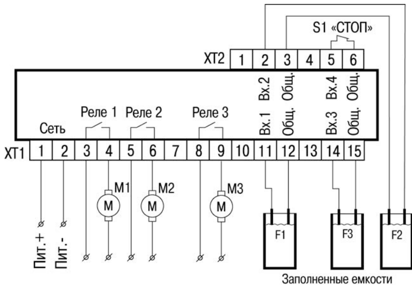
Рисунок В.4 – Схема подключения ОВЕН САУ-У-Н для выполнения алгоритма 06 М1–М3 – насосы; F1–F3 – кондуктометрические датчики уровня
