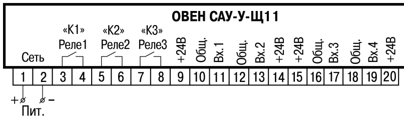
Рисунок Б.2 – Схема подключения ОВЕН САУ-У-Щ11
