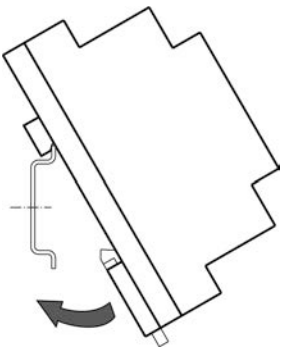
Рисунок 6.3 – Монтаж прибора с креплением на DIN-рейку
