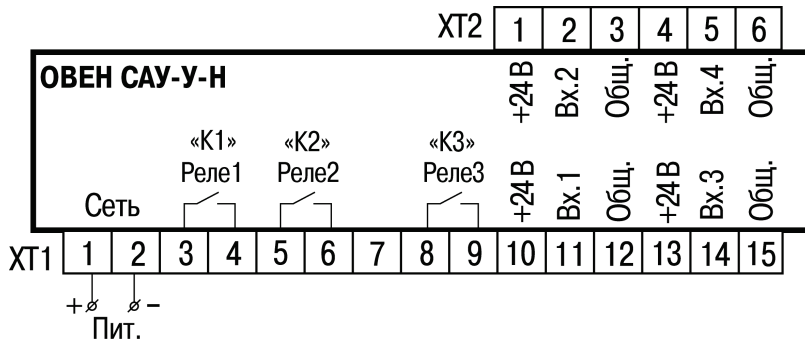
Рисунок Б.1 – Схема подключения ОВЕН САУ-У-Н
