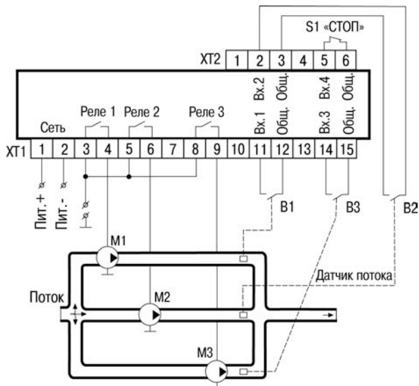
Рисунок В.11 – Схема подключения ОВЕН САУ-У-Н для выполнения алгоритма 14 М1–М3 – насосы; F1–F3 – кондуктометрические датчики уровня; В1–В3 – датчики потока
