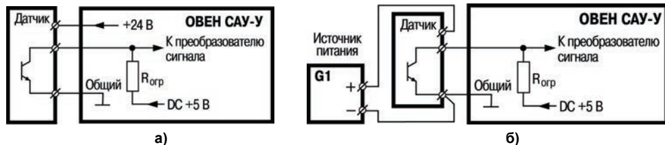
Рисунок 3.8 – Схема подключения датчиков с выходными ключами n-p-n типа: а) с питанием от прибора; б) с питанием от внешнего источника
