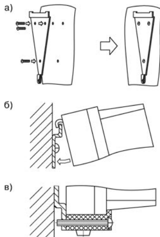
Рисунок 6.1 – Монтаж прибора настенного крепления
