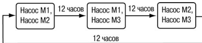
Рисунок В.10 – Порядок работы насосов в режиме «два из трех»
