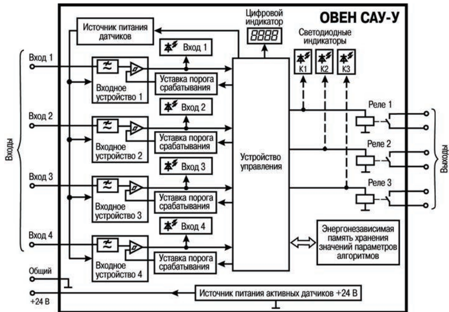
Рисунок 3.4 – Функциональная схема
