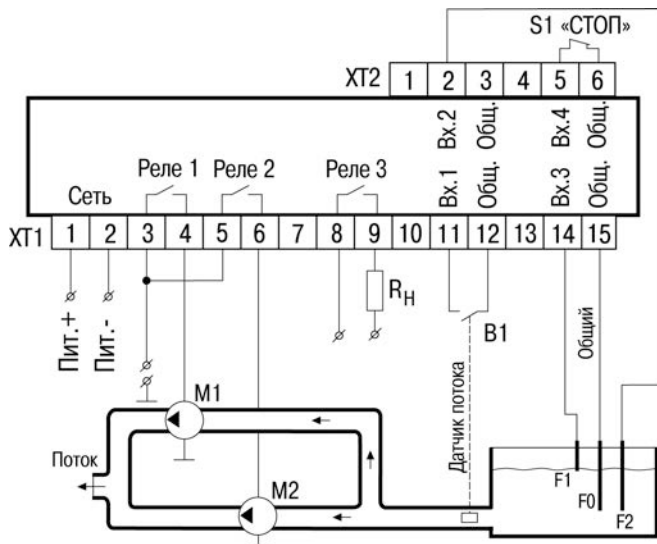
Рисунок В.12 – Схема подключения ОВЕН САУ-У-Н для выполнения алгоритма 16 M1 и M2 – насосы; R H – сигнализатор аварии или дополнительный насос; B1 – датчик потока; F1, F2 – кондуктометрические датчики уровня
