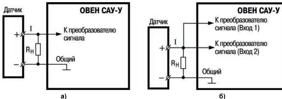
Рисунок 3.9 – Схема подключения нагрузочного резистора для токового датчика:
