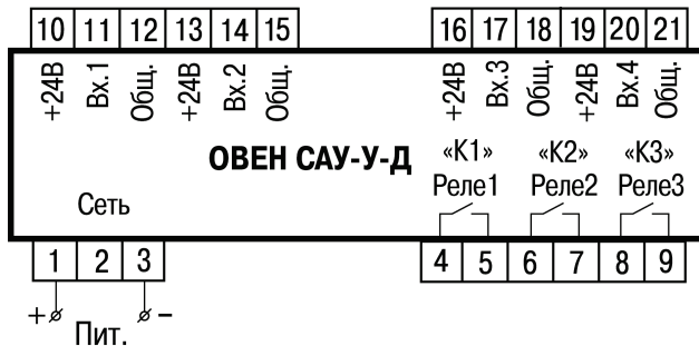
Рисунок Б.3 – Схема подключения ОВЕН САУ-У-Д
