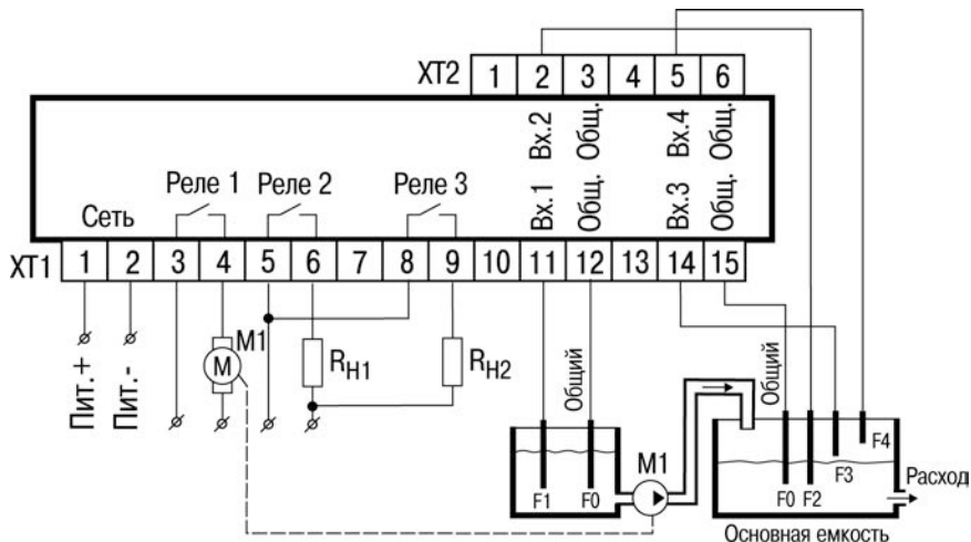
Рисунок В.15 – Схема подключения ОВЕН САУ-У-Н для выполнения алгоритма 20 M1 – насос; F1–F4 – кондуктометрические датчики уровня; R Н1 – сигнализатор недостаточного количества жидкости в откачиваемой емкости (сухой ход насоса); R Н2 – сигнализатор аварии (перелив в основном баке)
