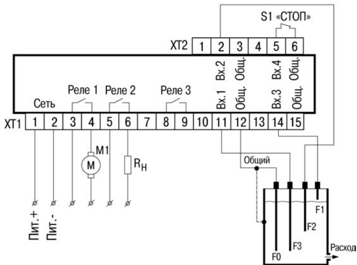
Рисунок В.1 – Схема подключения ОВЕН САУ-У-Н для выполнения алгоритма 01 M1 – исполнительное устройство (насос, электромотор, клапан или др.); Rn – сигнализатор (звонок, сирена, лампа или блокирующий контактор); F1–F3 – кондуктометрические датчики уровня
