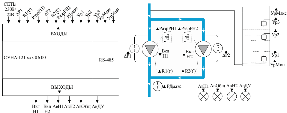
Рисунок 2.1 – Схема объекта управления
