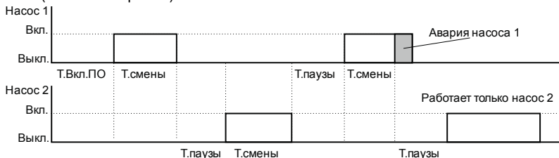
Рисунок 3.1 – Диаграмма переключения насосов
