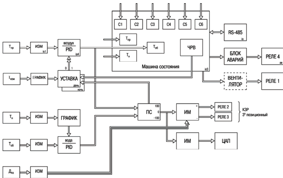
Рисунок 4.2 – Блок-схема работы прибора
