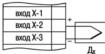
б) термопара
