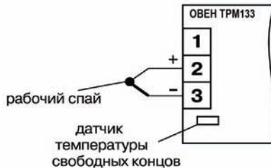
Рисунок 3.4 – Схема подключения ПТ
