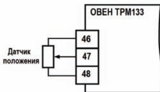
Рисунок 3.6 – Схема подключения резистивного датчика положения
