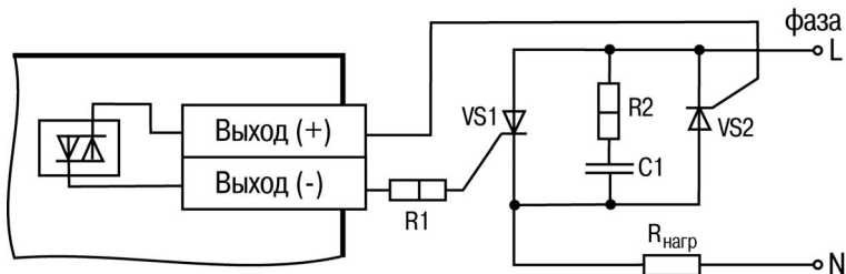
Рисунок Б.12 – Схема подключения нагрузки к ВЭ типа «С» двух тиристоров, подключенных встречно-параллельно ( R_2=47... 68 \text{ Ом} , C_1=0.1\text{мкф}\times 630 \text{ В} )
