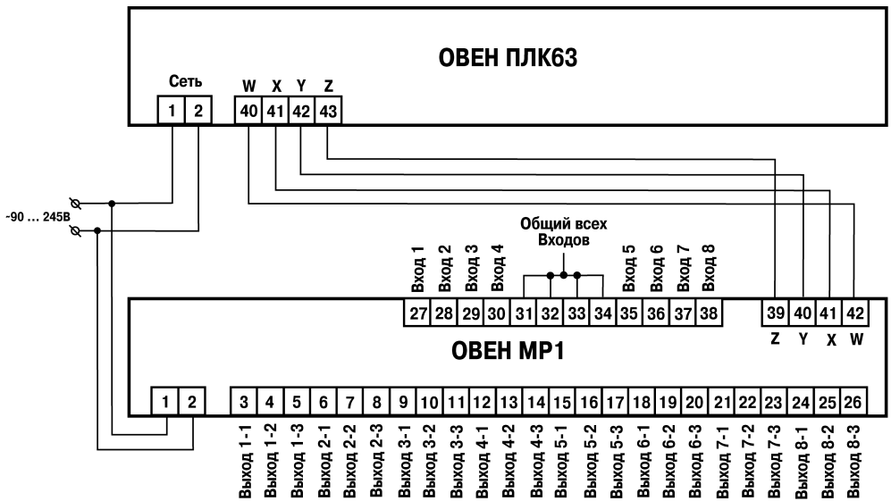
Рисунок Б.15 – Схема подключения модуля ОВЕН МР1 к контроллеру
