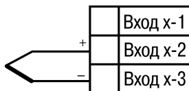
Рисунок Б.6 – Схема подключения преобразователя термоэлектрического (термопары)
