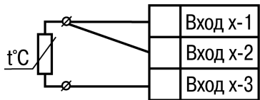
Рисунок Б.2 – Подключение термопреобразователя сопротивления или резистивного датчика по трехпроводной схеме
